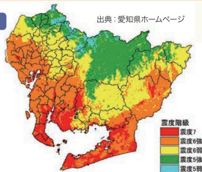
震度分布
